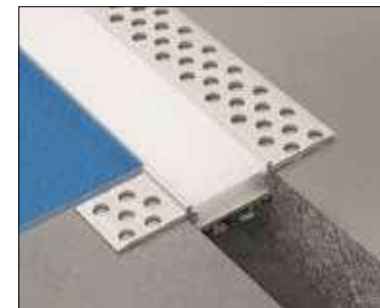
Incasso a raso F 206 L79xH14mm - Luce 31,5mm [100-300cm] Cartongesso ESCLUSO
